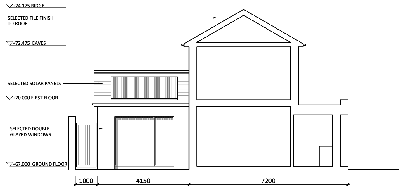
HOUSETYPE 3A SECTION AA
